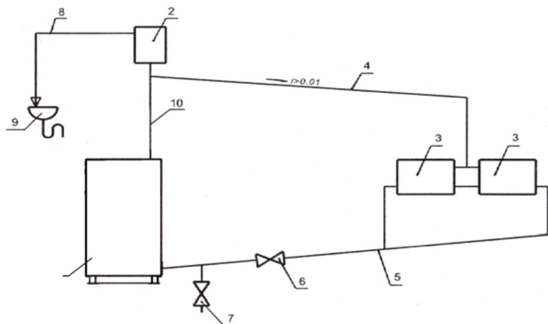
Рис. 5 Схема открытой системы отопления
